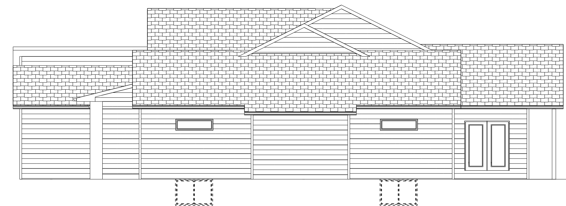
RIGHT ELEVATION
